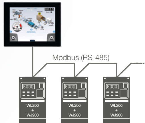
Direktkommunikation Hitachi-HMI an WL200/WJ200
