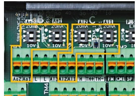
2 Analogeingang- und 2 Analogausgänge mittels DIP-Schalter umschaltbar für 0-10V- oder 0-20mA-Signale
